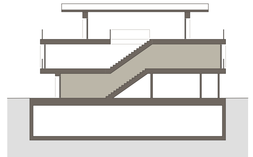
GEBÄUDESNITT
