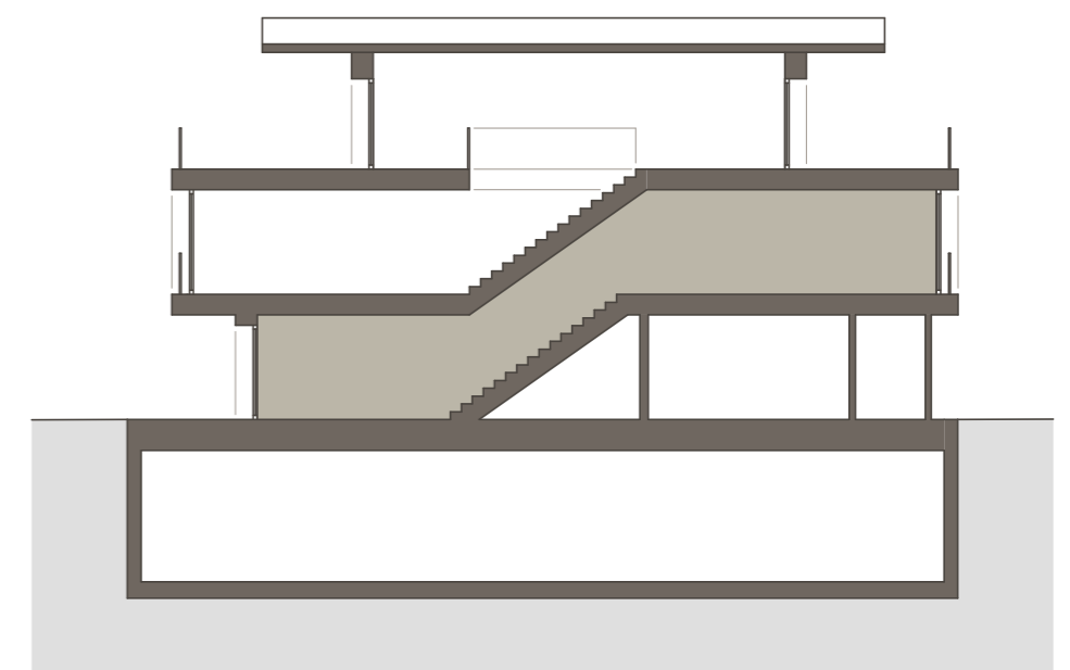
GEBÄUDESCHNITT
