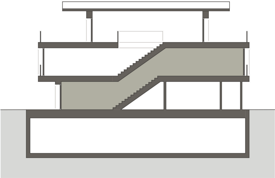
GEBÄUDESCHNITT
